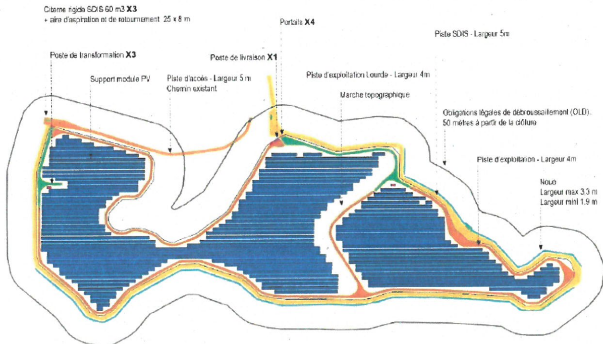
Figure 2: Plan de masse de la centrale photovoltaïque (Source : Permis de construire)
